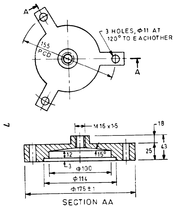
FIG. 4 DRAINAGE CAP
