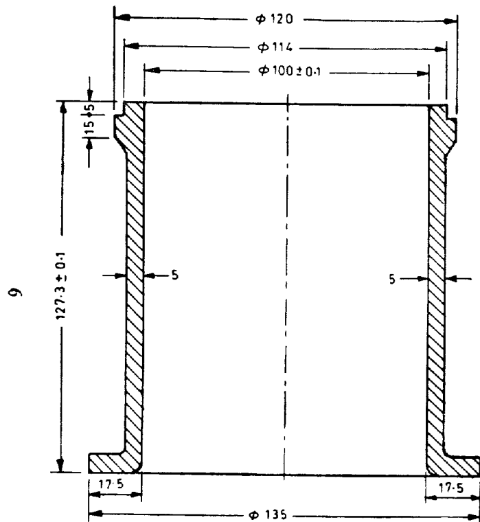
FIG. 2 MOULD
