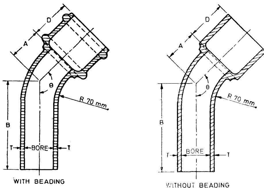
FIG. 3 PLAIN BEND
